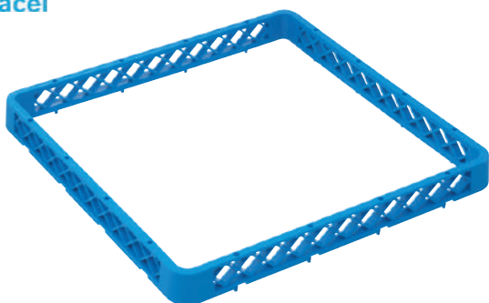
12630 RIALZO PER BASE UNIVERSALE BLU APERTO cm 50x50 - Dimensione interna cm 47,6x47,6 H 4,5
